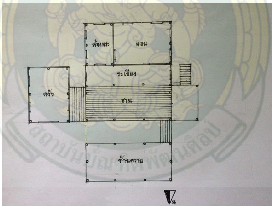
ภาพที่ 93 แปลนบ้านทรงไทย
