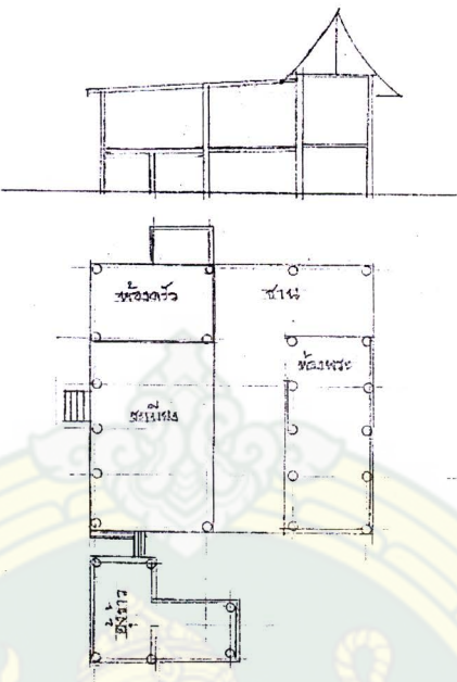
ภาพที่ 65 ผังบ้านนางฉลอง จันทรเกตุเลียด
